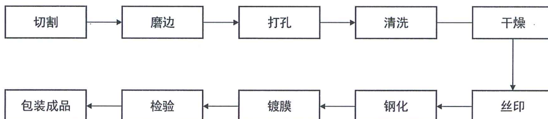
图 3-1 微波炉门板玻璃产品主要生产工艺流程图
